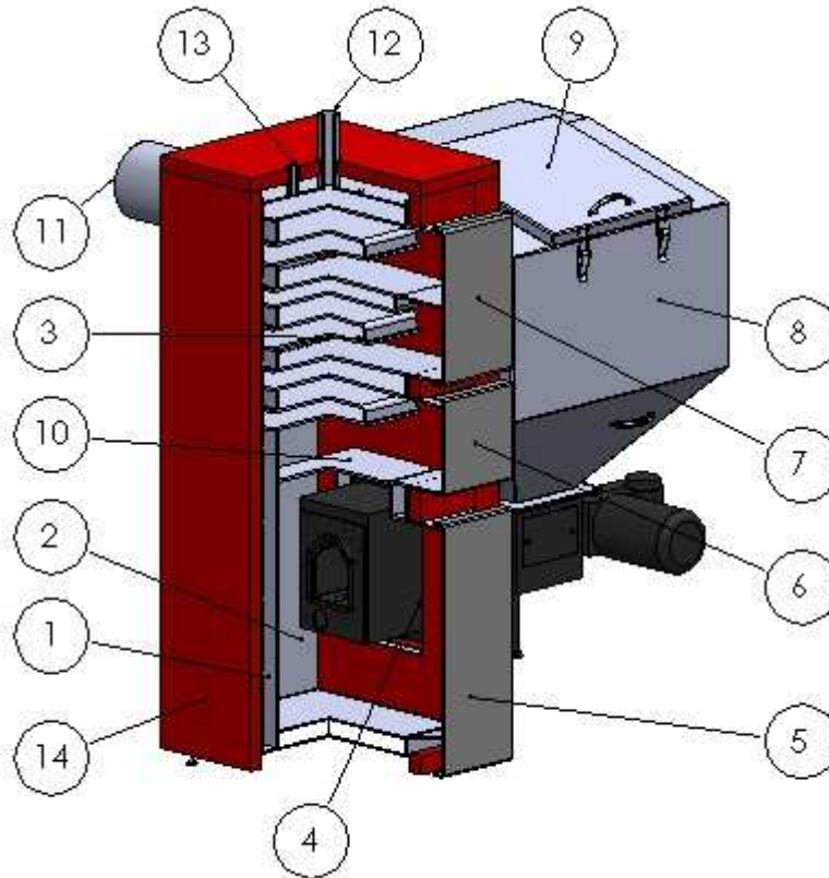
Rys.1. Kocioł "Technix (Uniwersal 5)"
